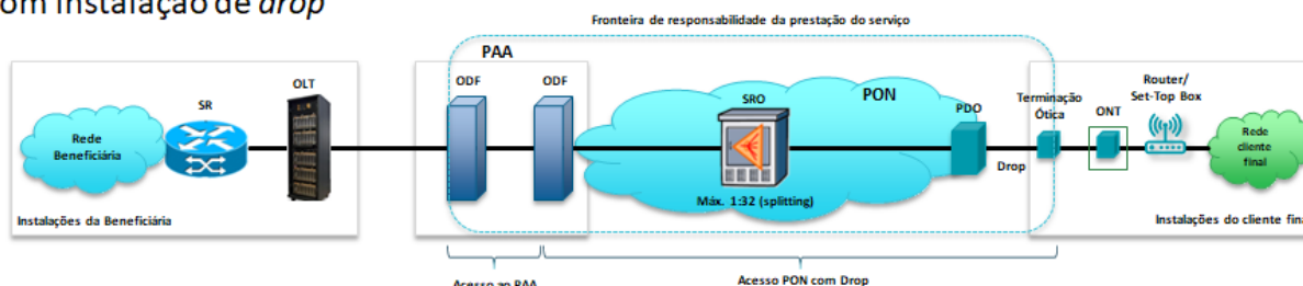
Figura 1. Arquitetura simplificada do serviço Acesso PON
